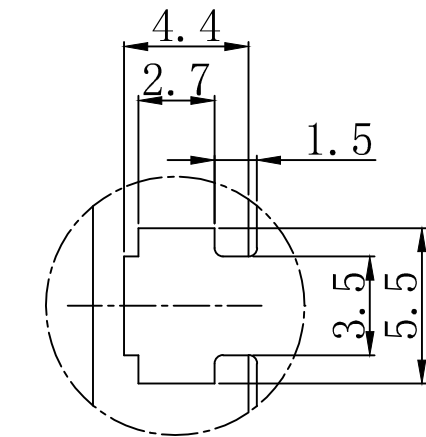
局部A 比例3:1 M3螺母凹槽，安装用
