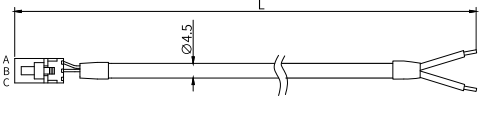
紧凑型通讯缆线外形尺寸图(4852C-P-3)
