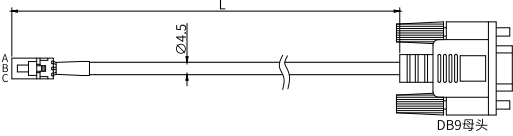
紧凑型通讯缆线外形尺寸图(LS-232-S-3)
