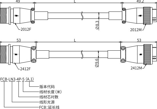
线光延长线外形尺寸图(FCB系列)
