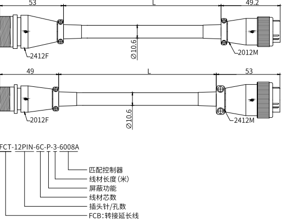
分时转接延长线外形尺寸图(FCT系列)
