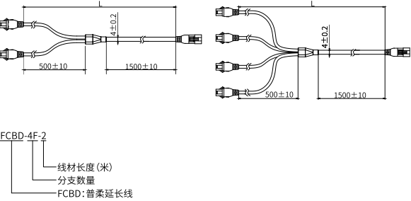
2分支/4分支普柔延长线外形尺寸图(FCBD系列)
