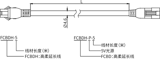
高柔延长线外形尺寸图(FCBDH/FCBDH-P系列)
