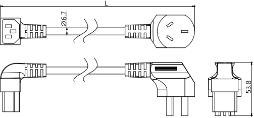
通讯缆线外形尺寸图(EAI-485-3-B)
