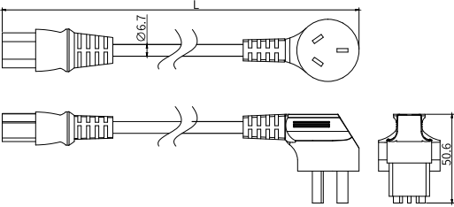
通讯缆线外形尺寸图(LS-232-3-B)
