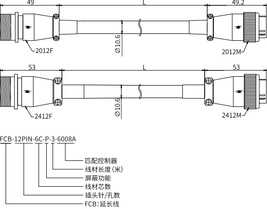
分时延长线外形尺寸图(FCB系列)
