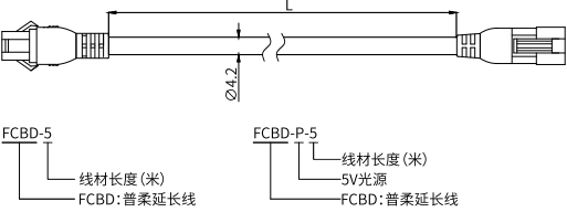
普柔延长线外形尺寸图(FCBD/FCBD-P系列)
