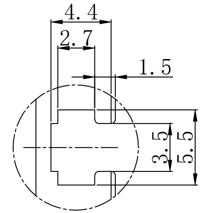
局部A 比例3:1 M3螺母凹槽，安装用
