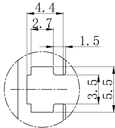
局部A 比例3:1 M3螺母凹槽，安装用
