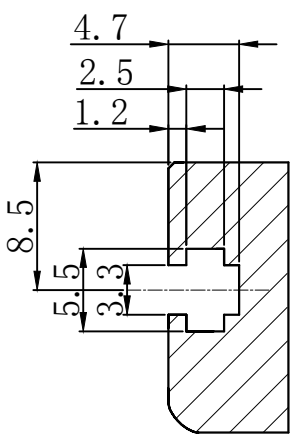
局部C 四面, M3螺母, 安装用 比例: 2: 1
