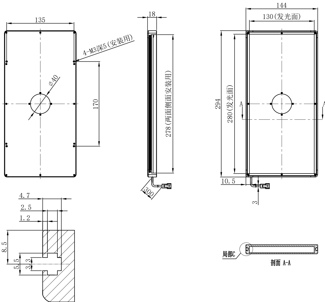
局部C 四面, M3螺母, 安装用
