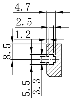
局部C 四面, M3螺母, 安装用
