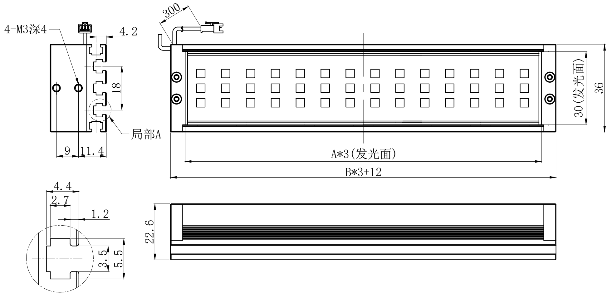
局部A 比例3:1 M3螺母凹槽，安装用
