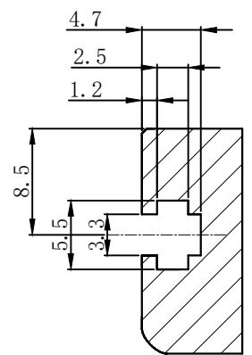
局部C 四面, M3螺母, 安装用 比例: 4: 1
